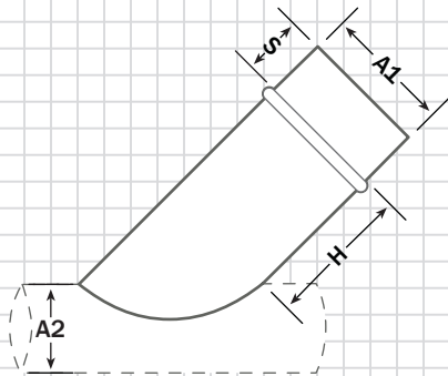
45° Lateral Tee (LT)
